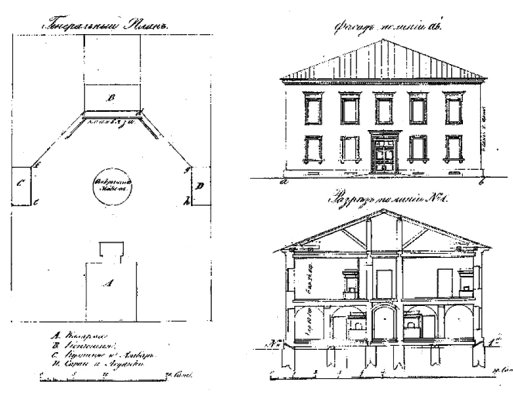
Проект постройки казармы и канцелярии жандармской команды в Керчи. 1844 г.
